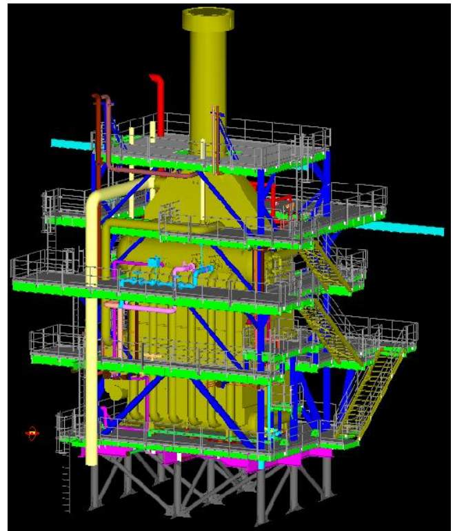
Tekla model of Cidade de Sao Mateus FPSO boiler module
